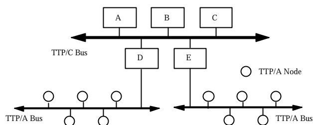
Figure 2: TTP/C and two TTP/A clusters.
