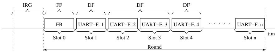
Figure 3: Layout of a TTP/A Round
